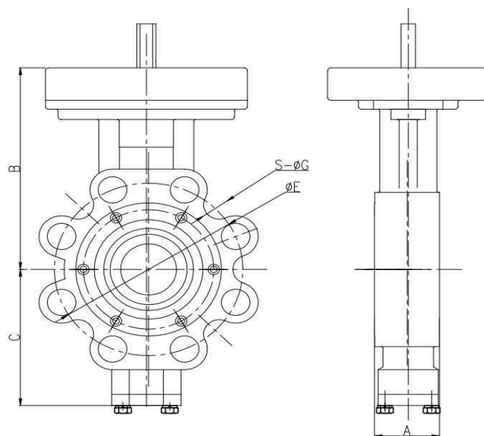
BFH200-CLASS 300 Unit:mm
