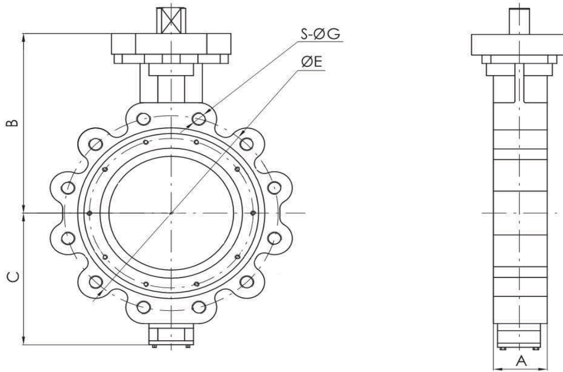
BFH400 - CLASS 300 Unit:mm
