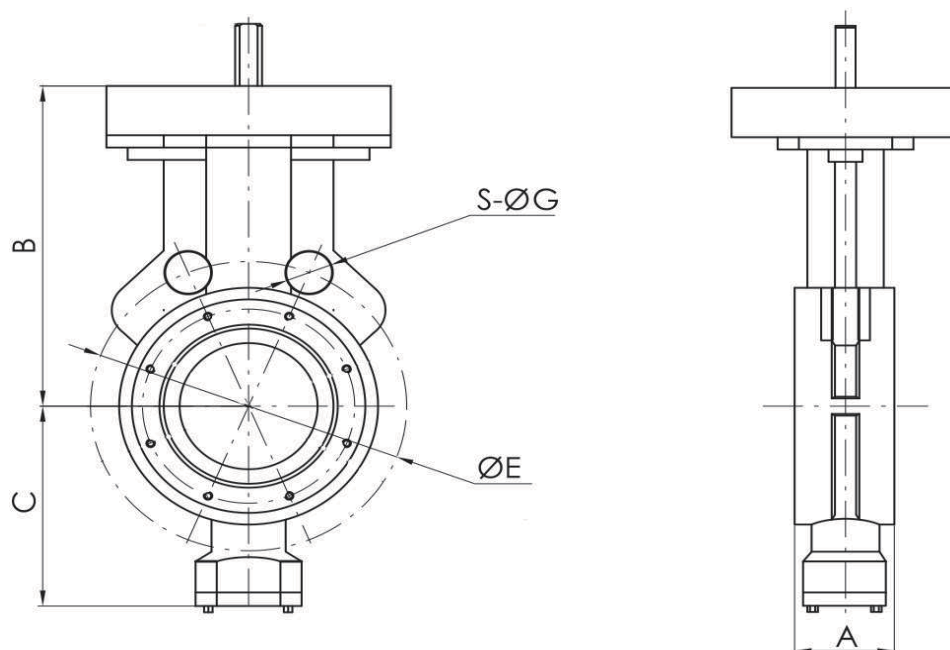
BFH200-CLASS 300 Unit:mm
